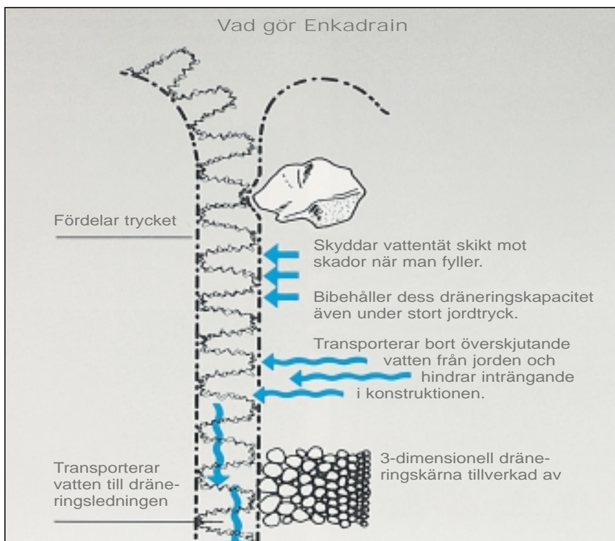
Uppbyggnaden säkrar en hög dräneringskapacitet och ett formidabelt membranskydd.
