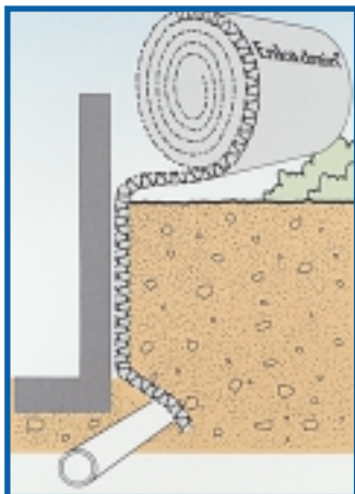
Användning av Enkadrain i samband med källarvägg
